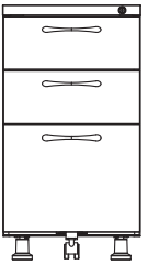
Box/Box/File Pedestal W 15 D 17-5/8 H 27-5/8 W 15 D 21-5/8 H 27-5/8
